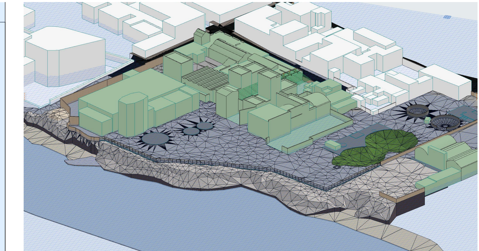
SOVRAPPOSIZIONE MODELLO BIM CON NUVOLE DI PUNTI - VISTA DALL'ALTO
