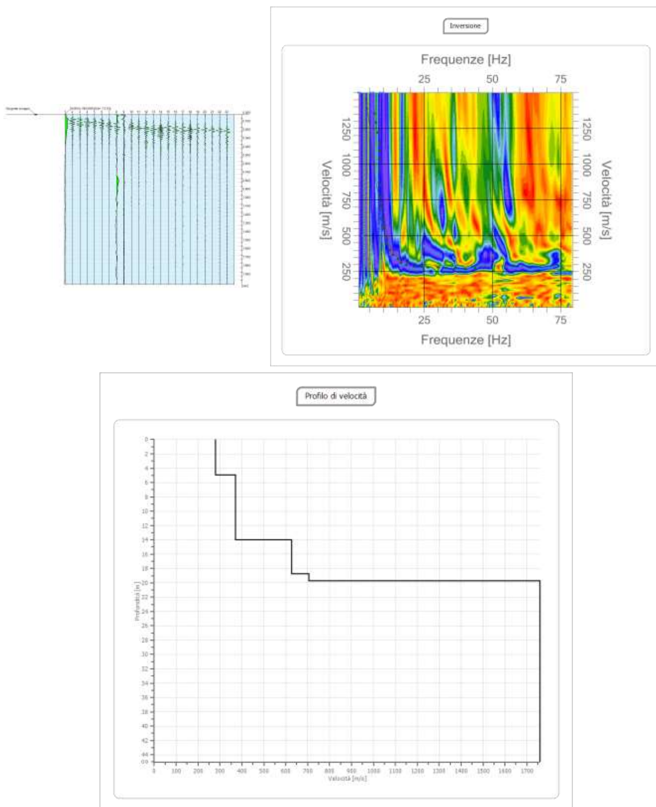
Fig. 54 - Spettro, sismogramma, sismostrato (Vs)
