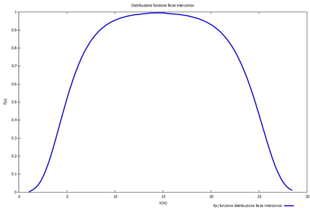
Fig. 43 – Diagrammi delle forze e distribuzione forze interconcreto
