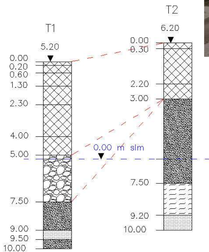
Fig. 20 – Foto e ricostruzione stratigrafica trivellazioni eseguite
