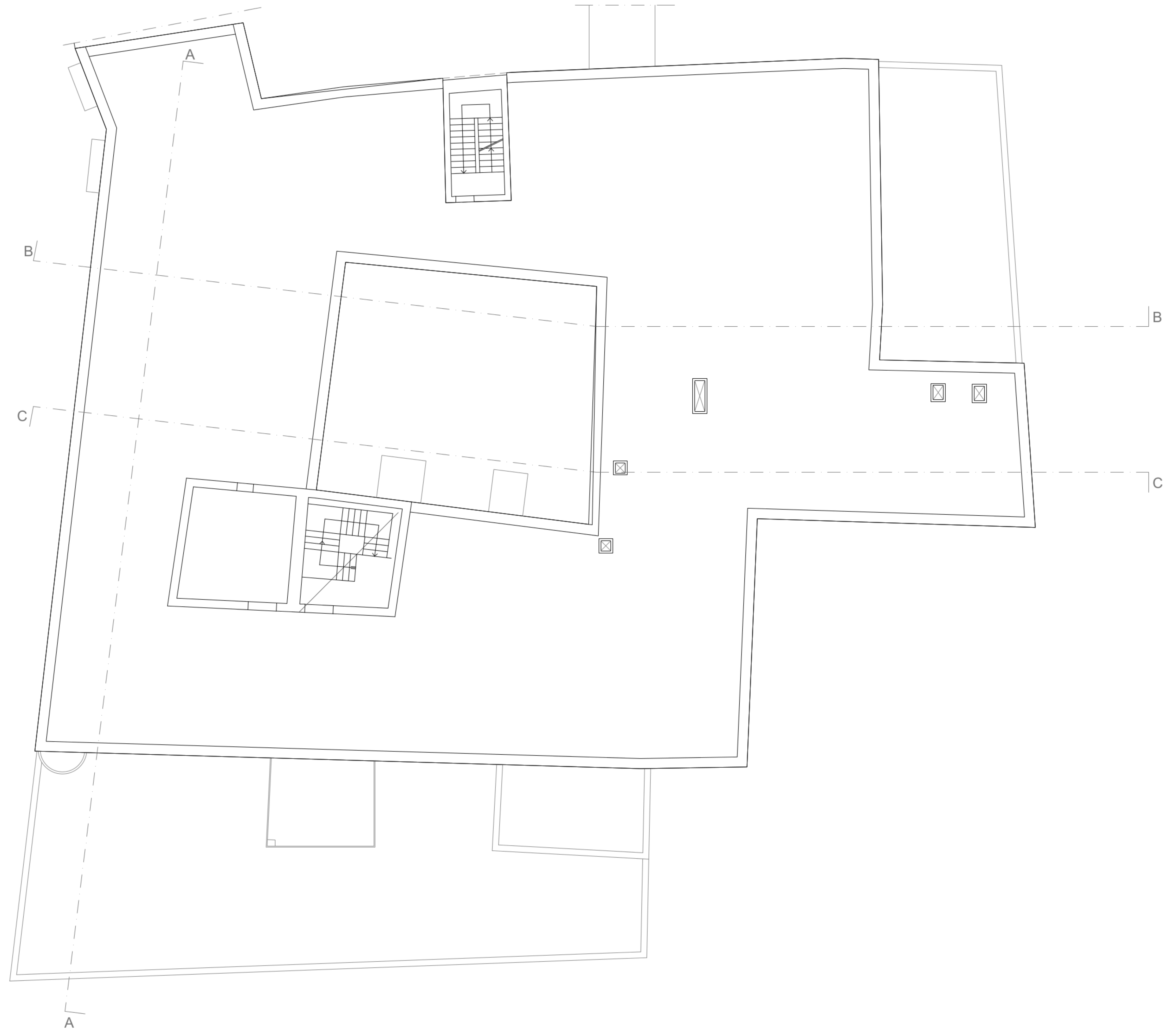
pianta coperture
