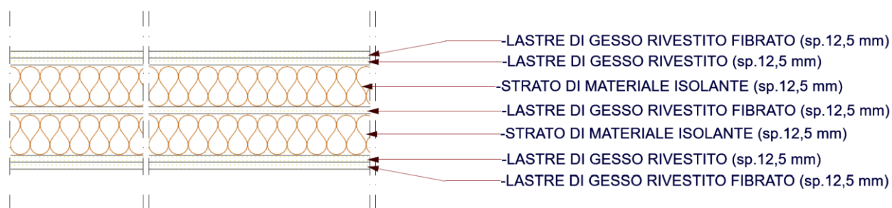
Figura 22: Particolare parete divisoria interna tra due appartamenti
