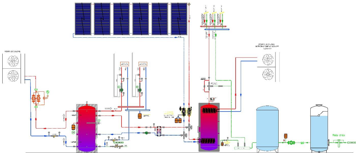
Figura 25 - schema centrale termica con riscaldamento con pdc ad integrazione solare termico, raffrescamento, produzione acs con solare termico ed integrazione pdc
