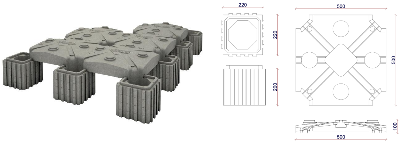
Figura 17: Vespaio ISO-AREATO in EPS
