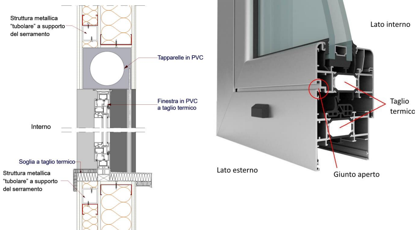
Figura 24: Sezione infisso ed esempio di infissi a taglio termico
