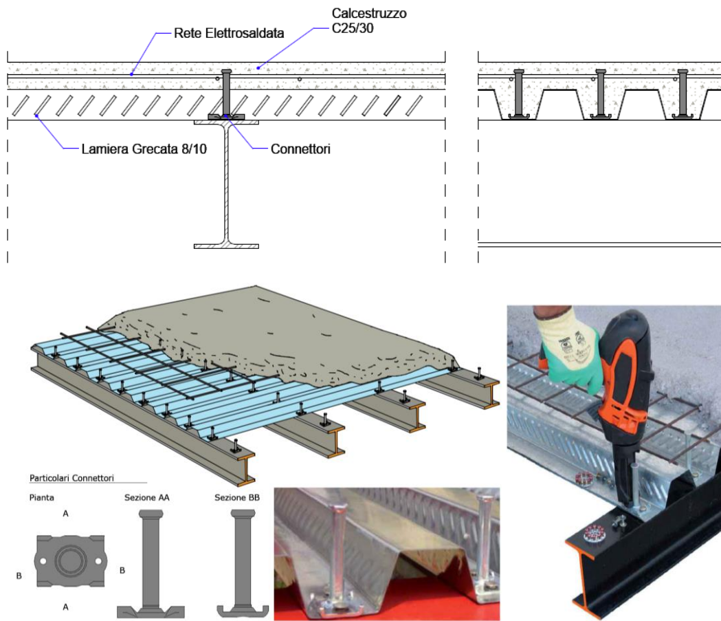
Figura 19: Particolare fissaggio lamiera grecata travi tramite connettori
