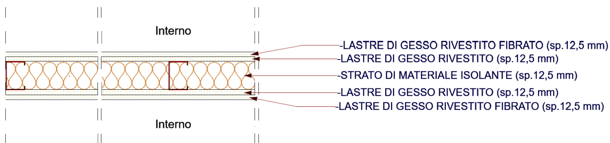
Figura 21: Particolare parete divisoria interna
