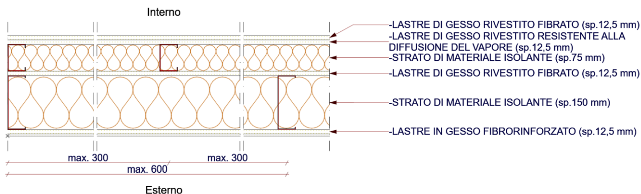
Figura 20: Particolare parete di tamponamento esterno
