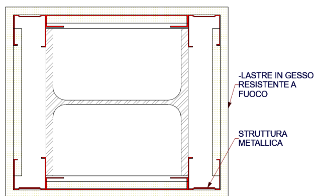
Figura 23: Particolare rivestimento pilastri con lastre in gesso resistenti al fuoco
