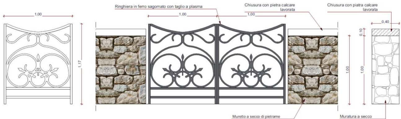
Figura 18: Particolare muratura a secco ringhiera
